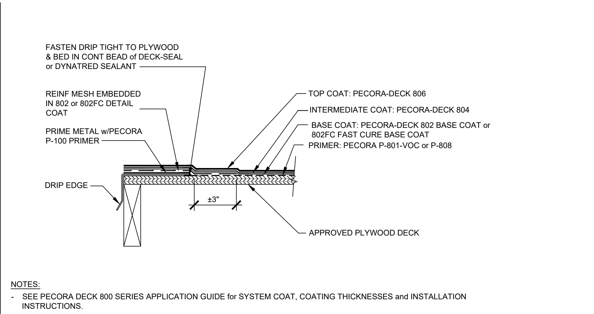
123B: PLYWOOD DRIP EDGE
